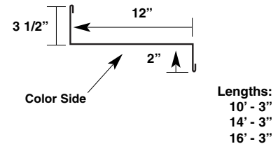
Valley Trim* (P-VF)
