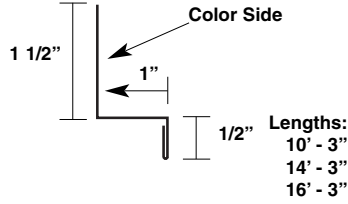
Rodent Guard (P-RG-72)
