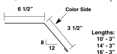
Gambrel Upper* (P-GU)
