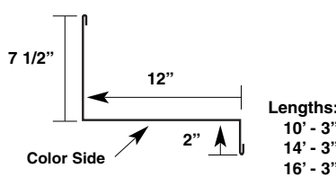
Gutter Apron* (P-GA)
