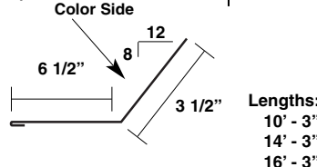
Gambrel Lower* (P-GL)
